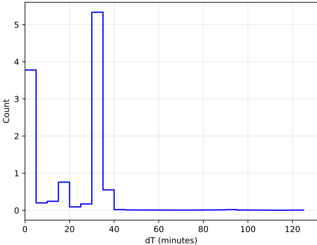
1e6 noroll_mjdp60_v3.4_10yrs WFD: DeltaT Histogram
