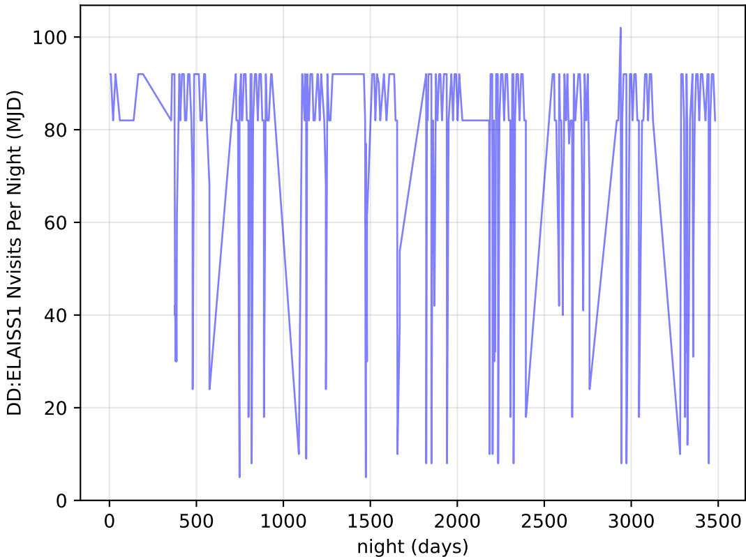
noroll_mjdp60_v3.4_10yrs all bands: DD:ELAISS1 Nvisits Per Night
