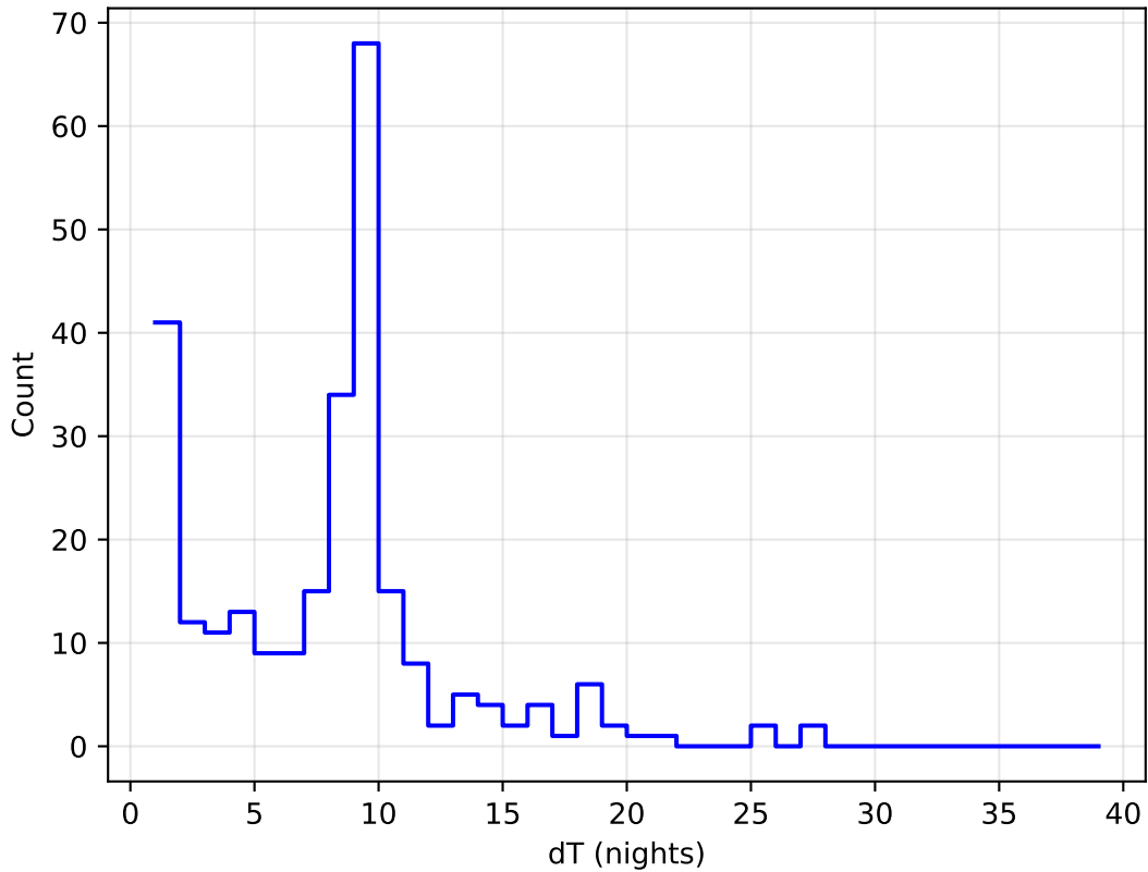
noroll_mjdp60_v3.4_10yrs all bands: DD:ELAISS1 Delta Nights Histogram
