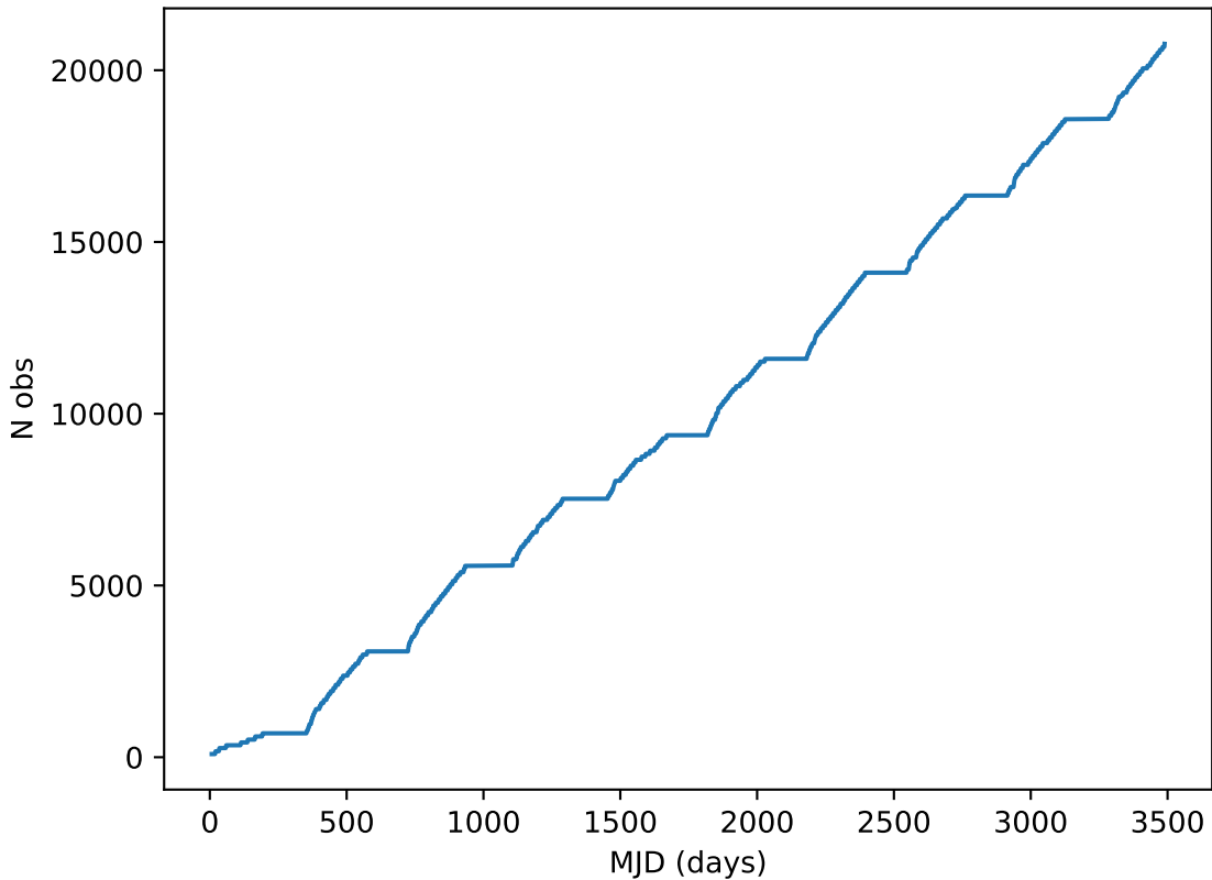
noroll_mjdp60_v3.4_10yrs all bands: DD:ELAISS1 Cumulative NVisits
