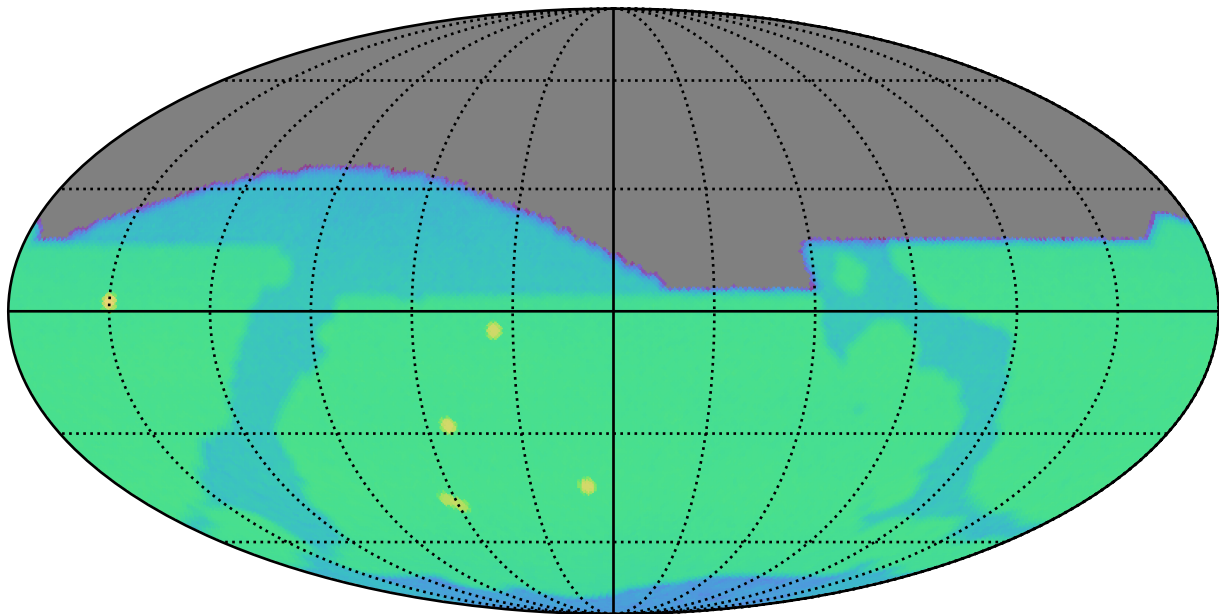
noroll_mjdp365_v3.4_10yrs i: SurfaceBrightLimit
