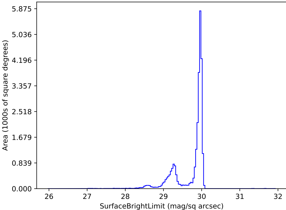
noroll_mjdp365_v3.4_10yrs i: SurfaceBrightLimit
