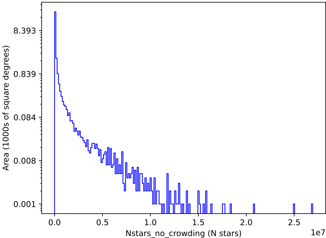
noroll_mjdp365_v3.4_10yrs i: Nstars_no_crowding
