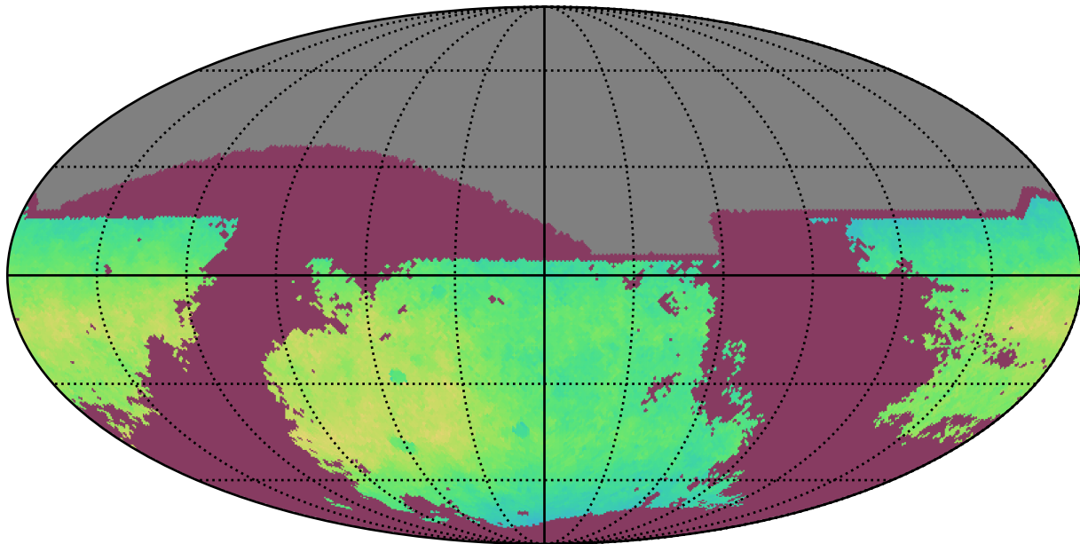
noroll_mjdp365_v3.4_10yrs i: NgalScale
