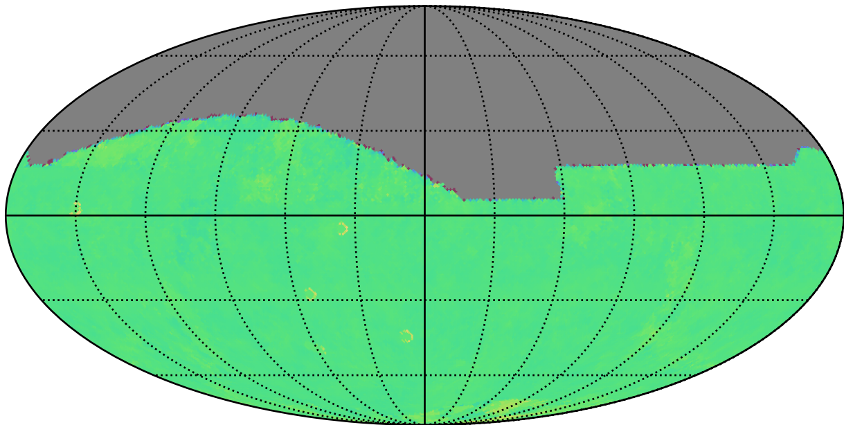
noroll_mjdp365_v3.4_10yrs z: Kuiper rotTelPos
