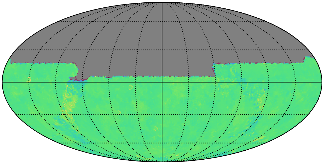
noroll_mjdp365_v3.4_10yrs u: Kuiper rotTelPos
