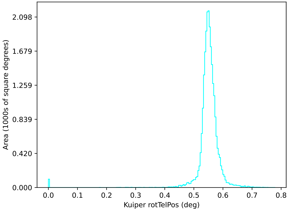
noroll_mjdp365_v3.4_10yrs u: Kuiper rotTelPos
