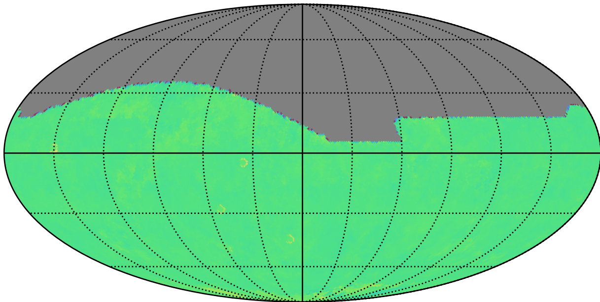
noroll_mjdp365_v3.4_10yrs r: Kuiper rotTelPos
