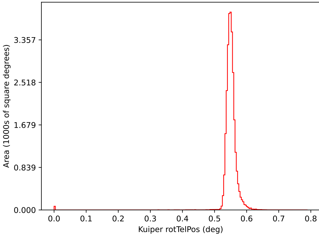
noroll_mjdp365_v3.4_10yrs i: Kuiper rotTelPos
