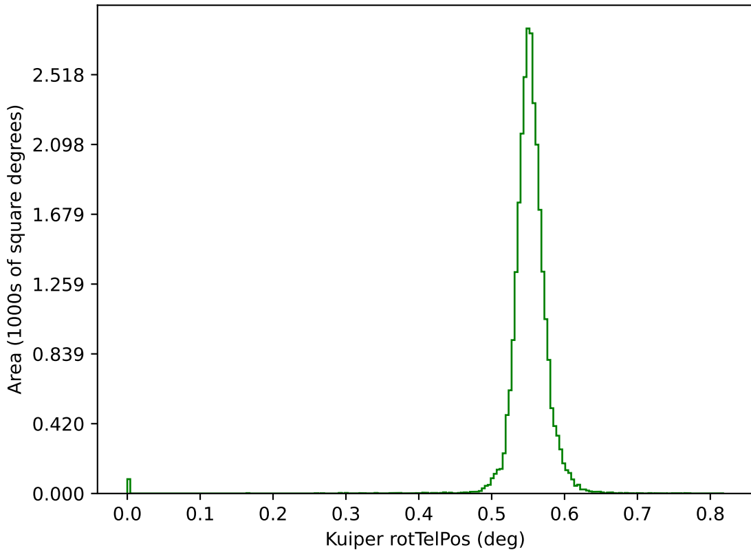
noroll_mjdp365_v3.4_10yrs g: Kuiper rotTelPos
