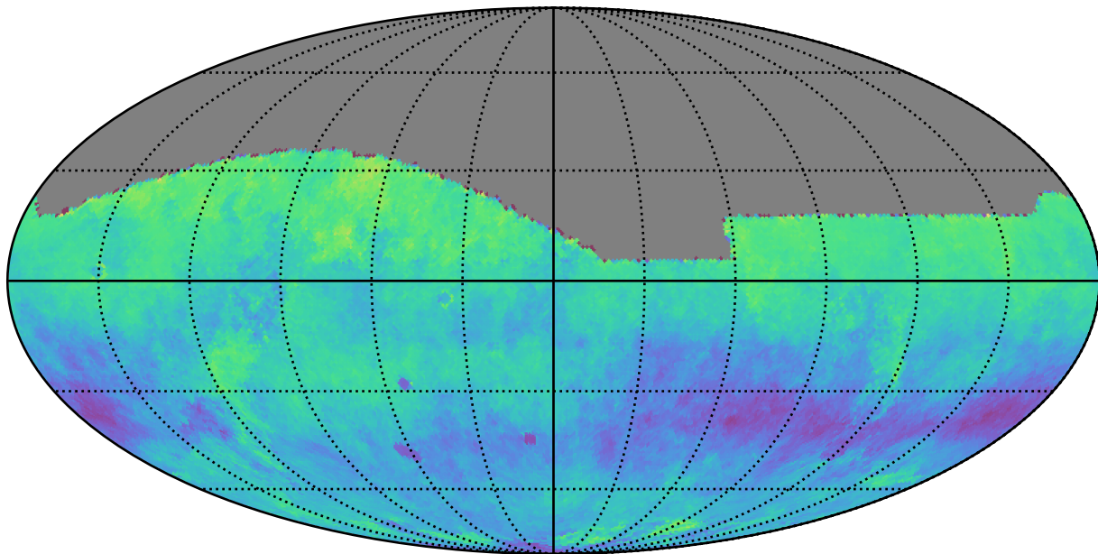
noroll_mjdp365_v3.4_10yrs z: Kuiper rotSkyPos
