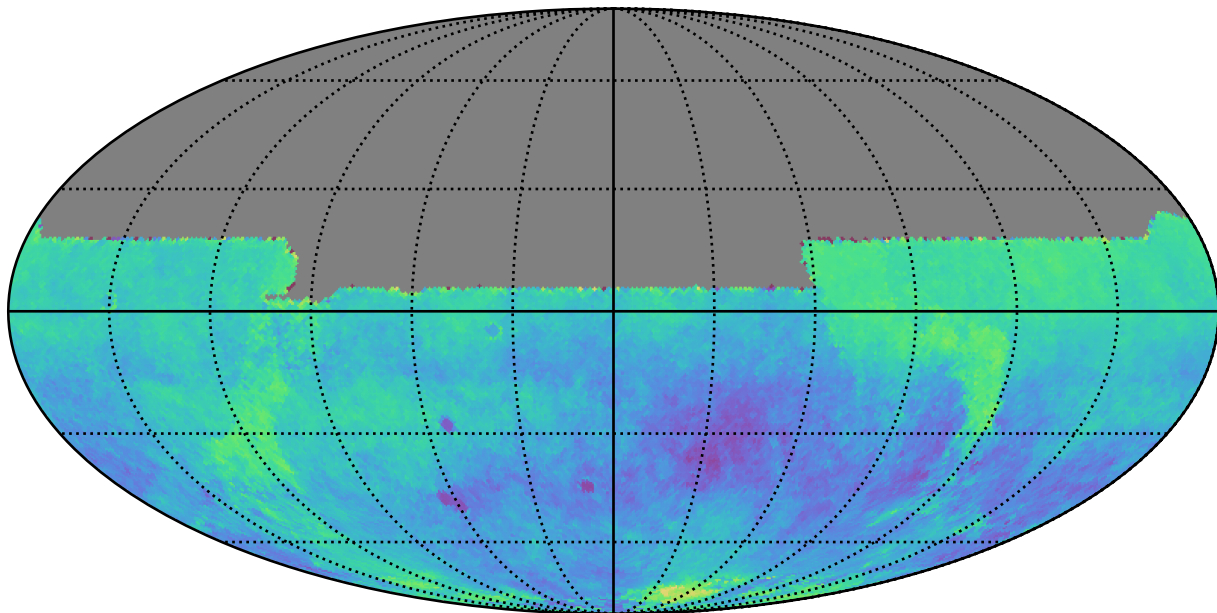
noroll_mjdp365_v3.4_10yrs y: Kuiper rotSkyPos
