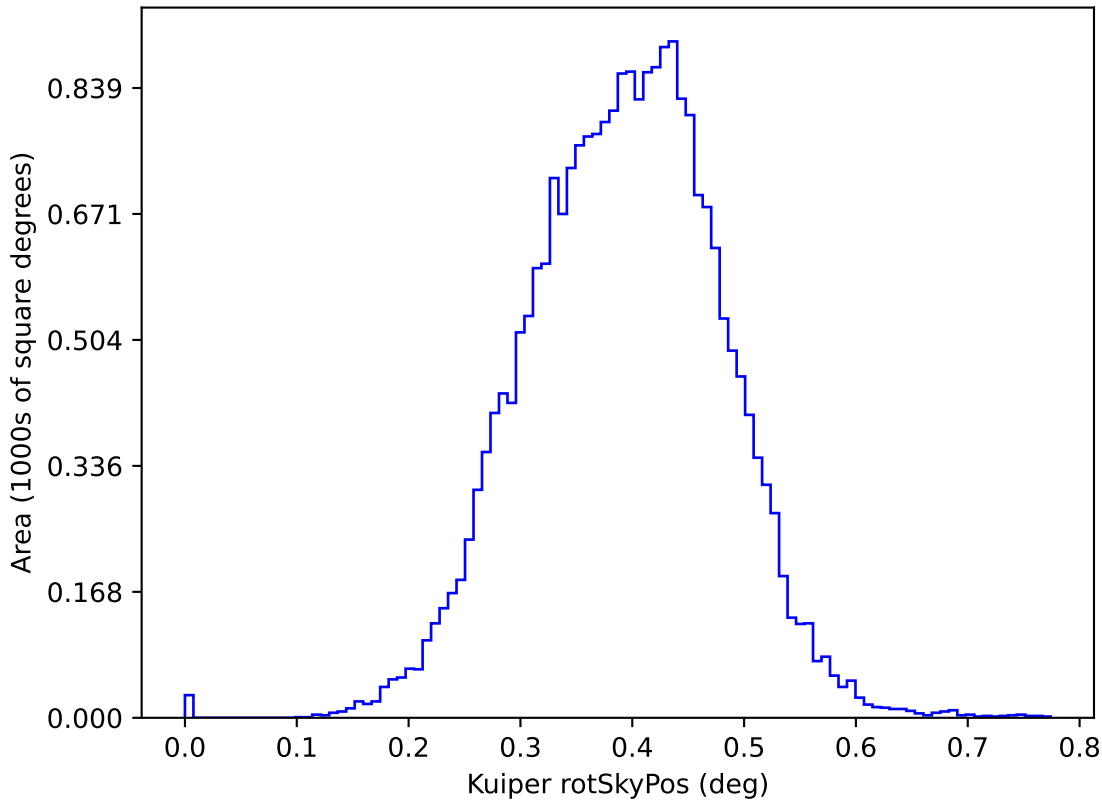
noroll_mjdp365_v3.4_10yrs y: Kuiper rotSkyPos
