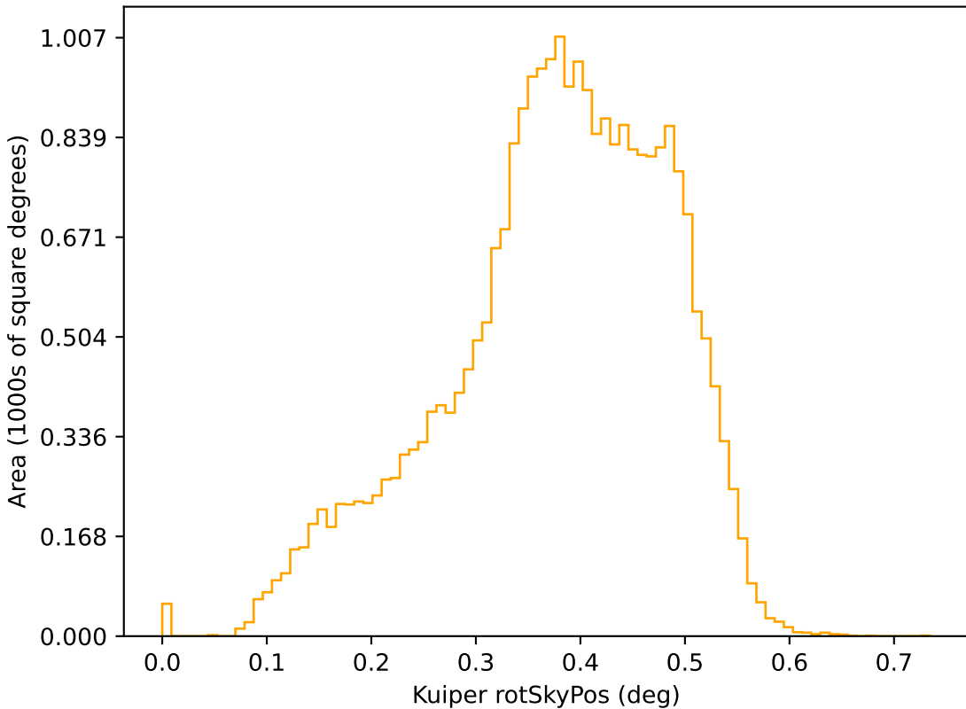
noroll_mjdp365_v3.4_10yrs r: Kuiper rotSkyPos
