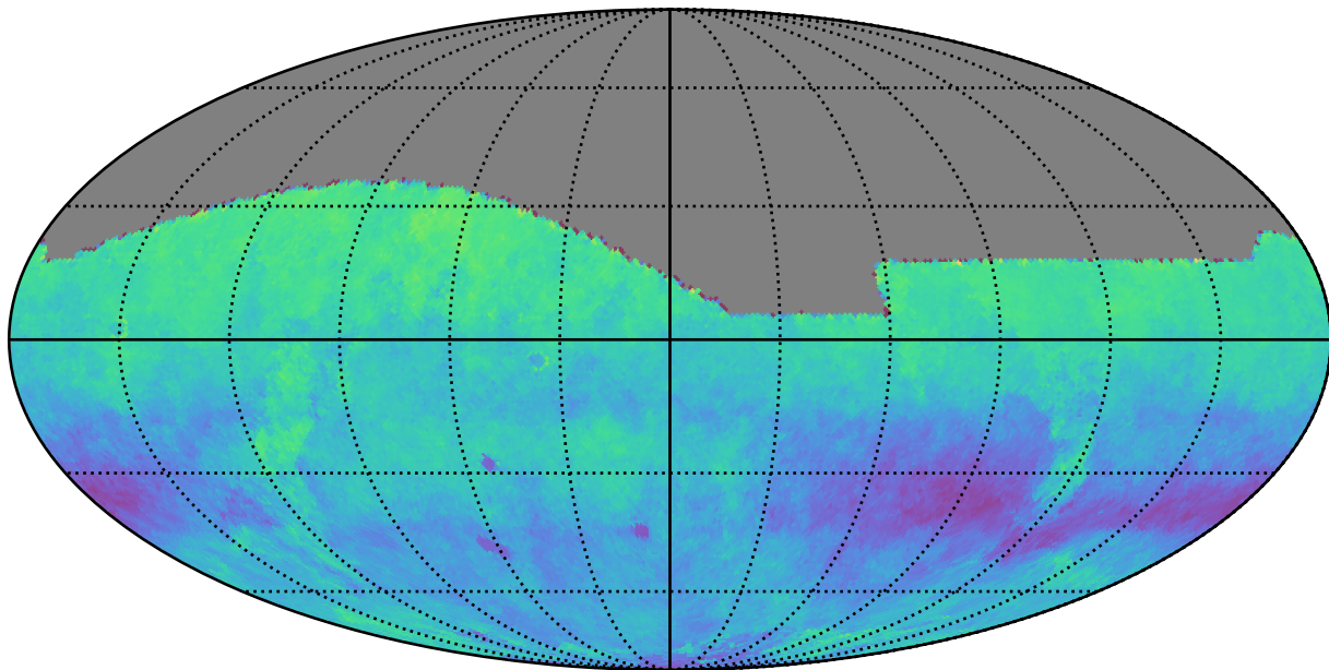
noroll_mjdp365_v3.4_10yrs i: Kuiper rotSkyPos
