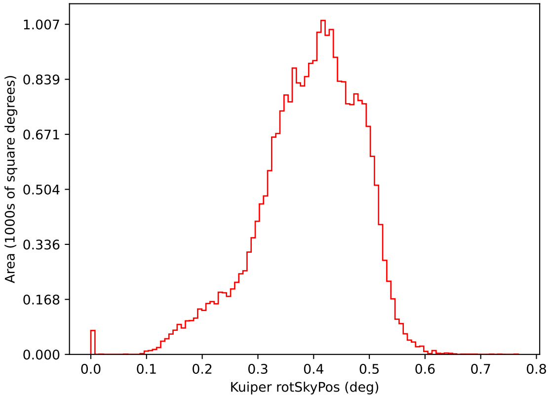
noroll_mjdp365_v3.4_10yrs i: Kuiper rotSkyPos
