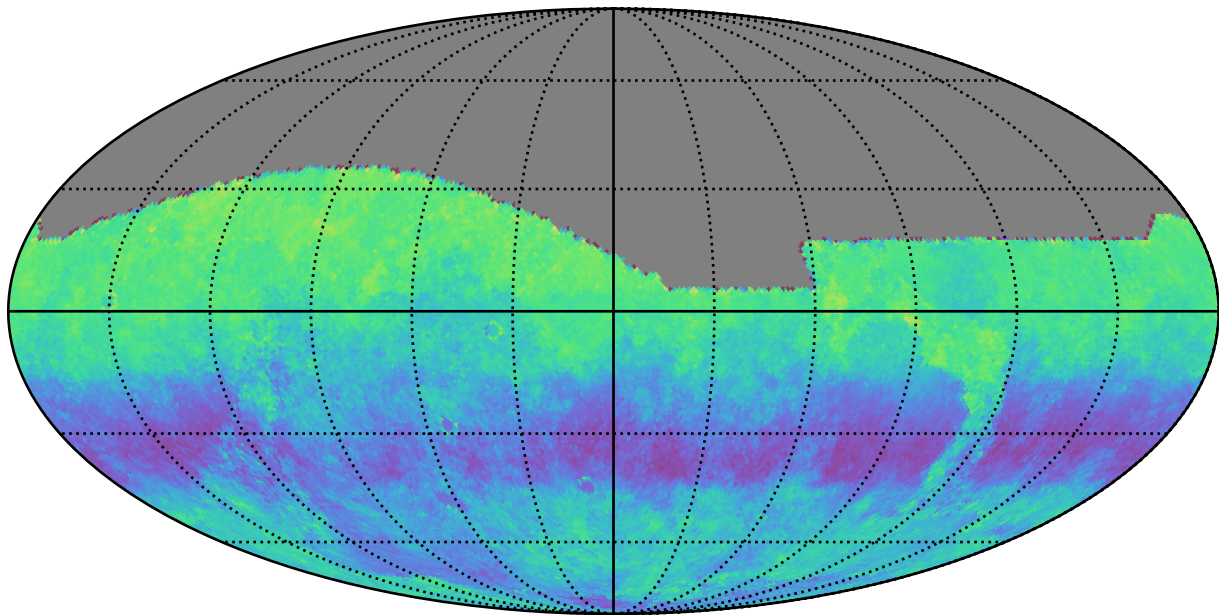
noroll_mjdp365_v3.4_10yrs g: Kuiper rotSkyPos
