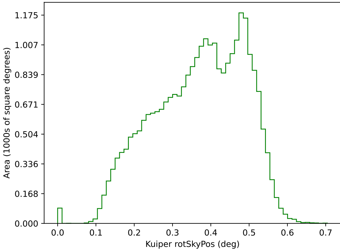
noroll_mjdp365_v3.4_10yrs g: Kuiper rotSkyPos
