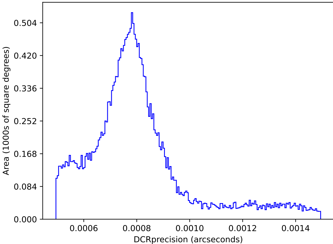
noroll_mjdp365_v3.4_10yrs : DCRprecision
