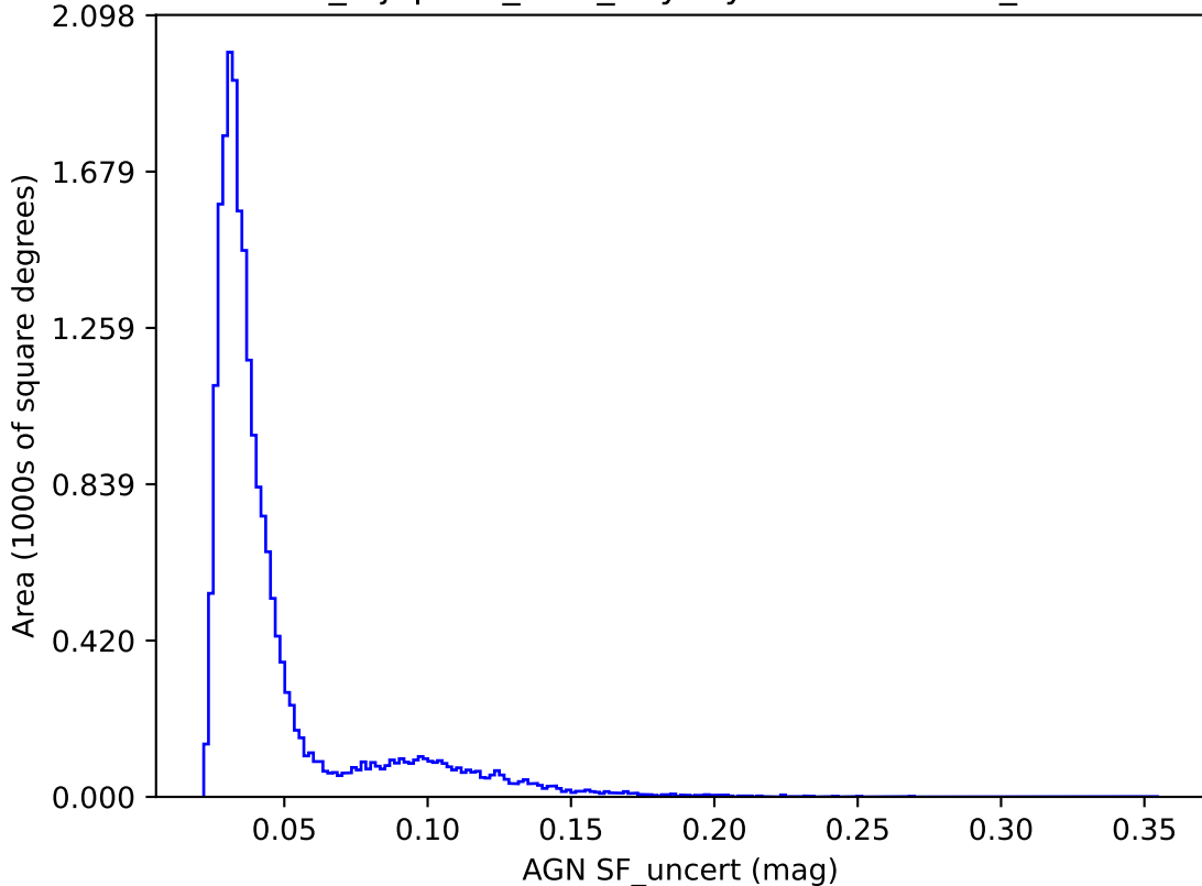
noroll_mjdp365_v3.4_10yrs y band: AGN SF_uncert
