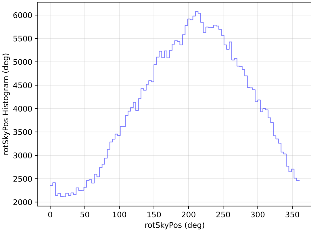
noroll_mjdp365_v3.4_10yrs All sky y band: rotSkyPos Histogram
