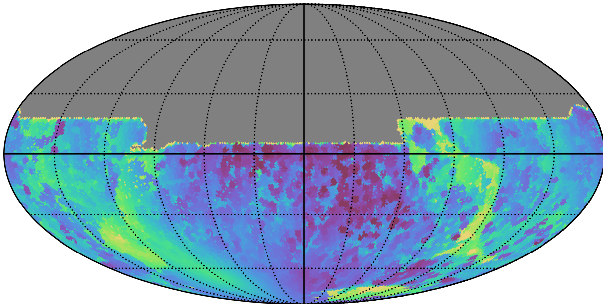
noroll_mjdp365_v3.4_10yrs All sky y band: Min solarElong
