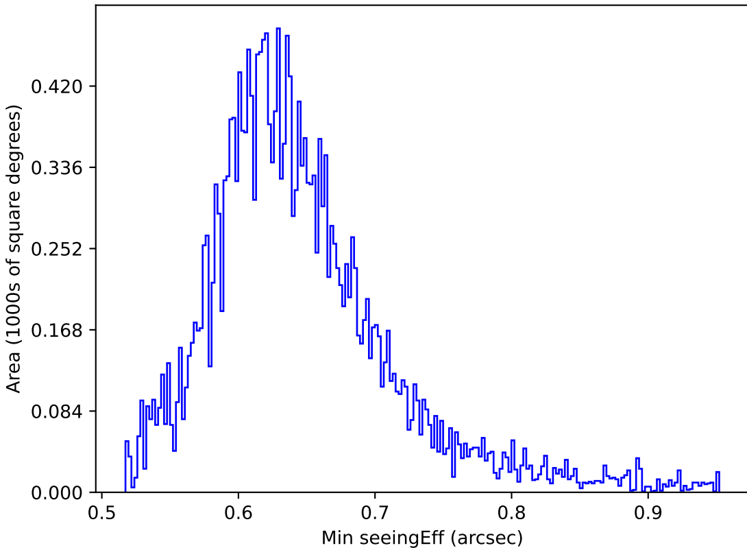
noroll_mjdp365_v3.4_10yrs All sky y band: Min seeingEff
