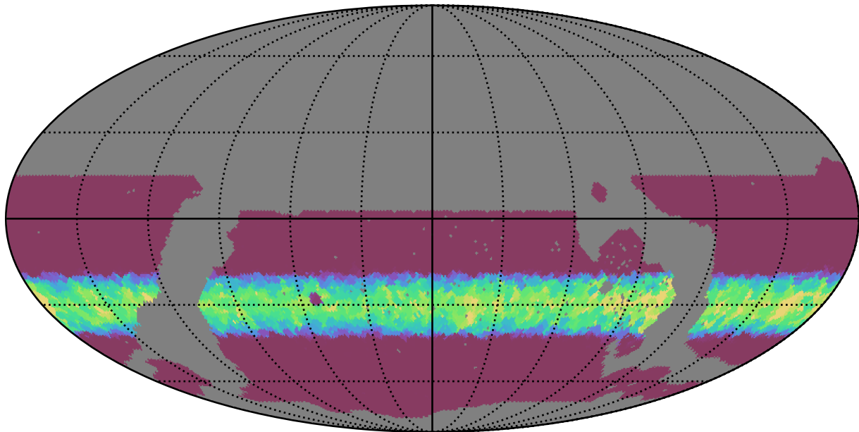
noroll_mjdp365_v3.4_10yrs WFD y band: Min normairmass
