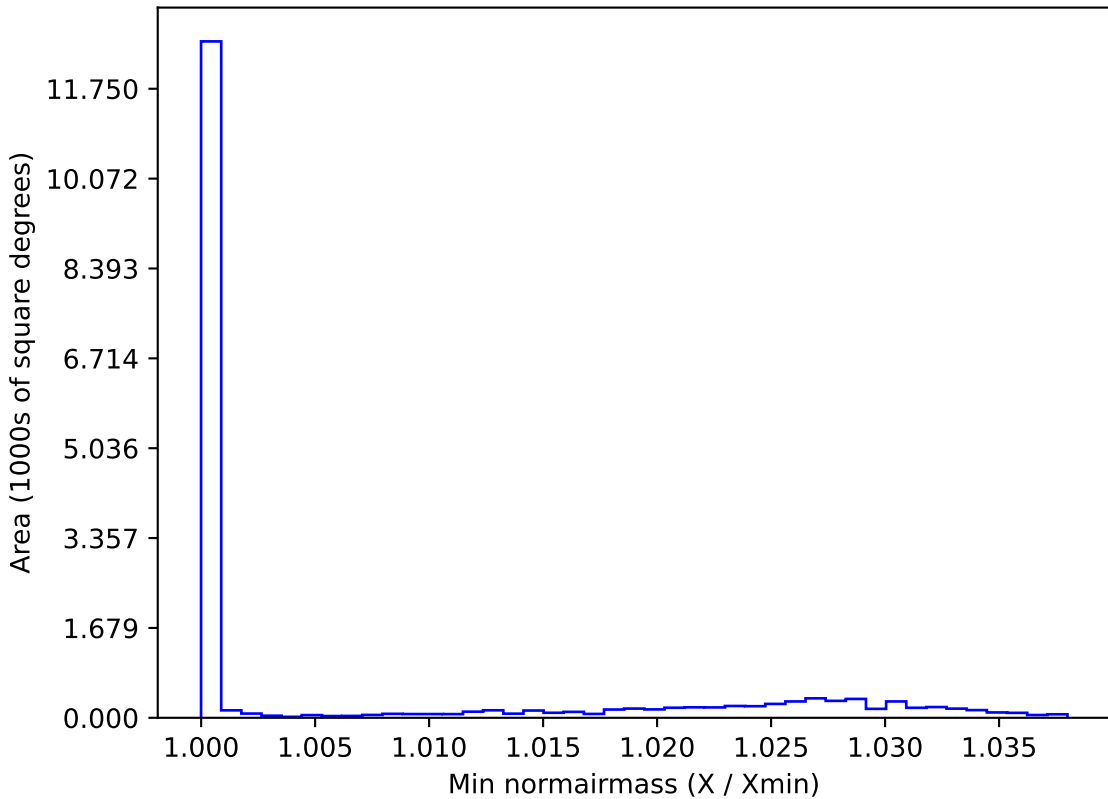
noroll_mjdp365_v3.4_10yrs WFD y band: Min normairmass
