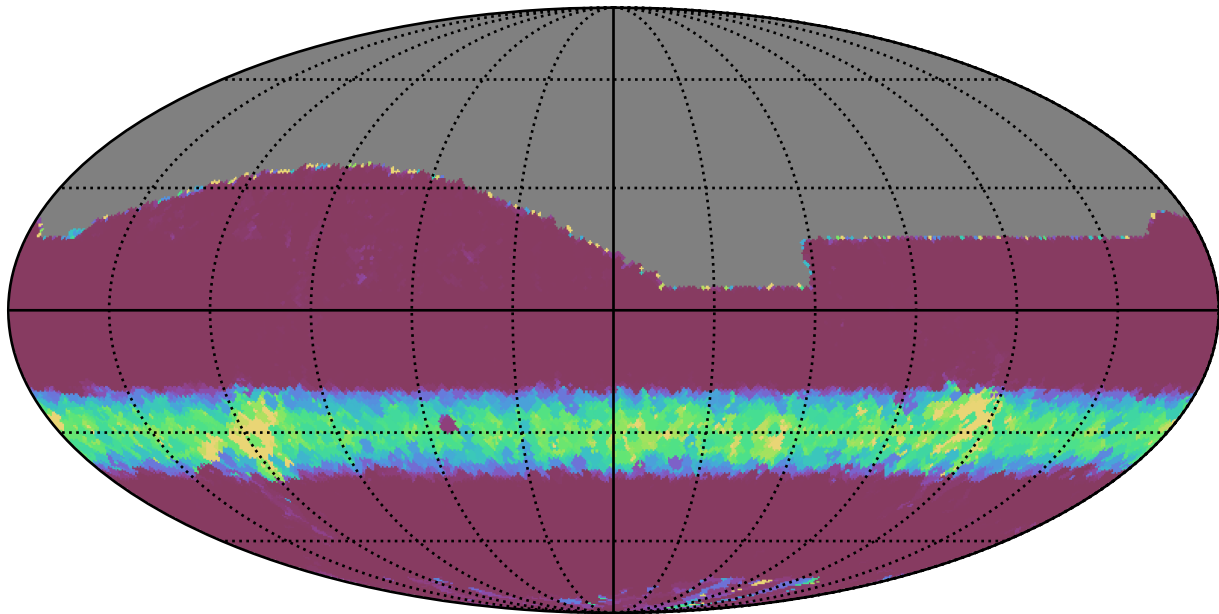
noroll_mjdp365_v3.4_10yrs All sky z band: Min normairmass
