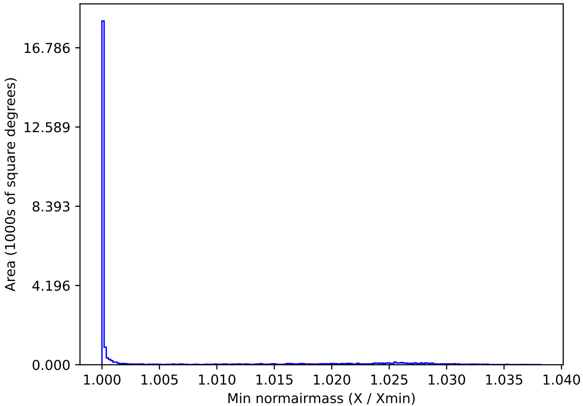
noroll_mjdp365_v3.4_10yrs All sky z band: Min normairmass
