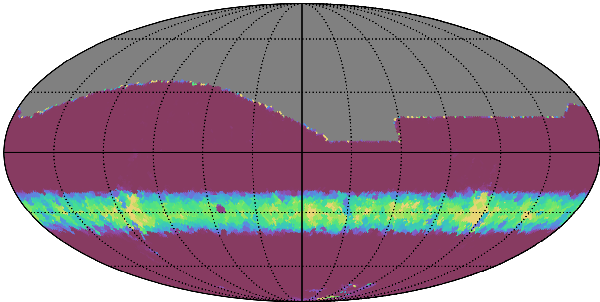
noroll_mjdp365_v3.4_10yrs All sky i band: Min normairmass
