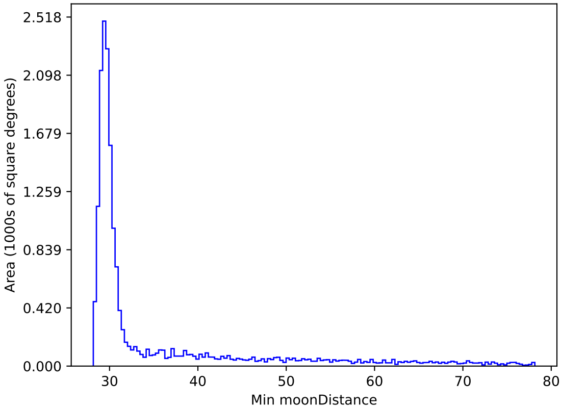
noroll_mjdp365_v3.4_10yrs WFD y band: Min moonDistance
