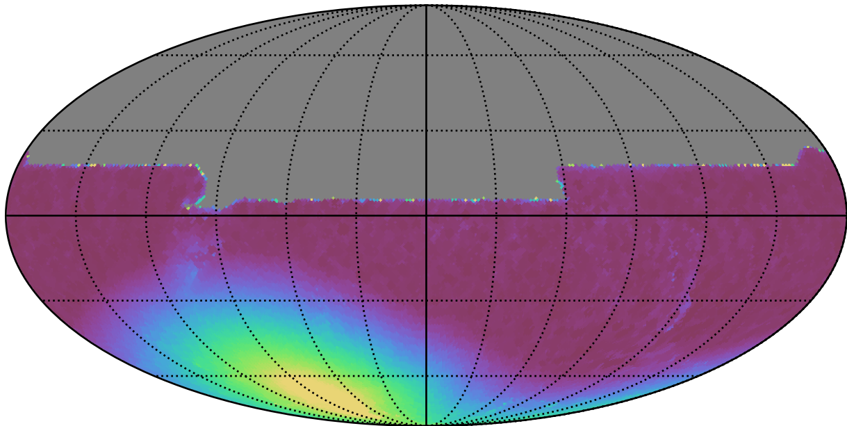
noroll_mjdp365_v3.4_10yrs All sky y band: Min moonDistance
