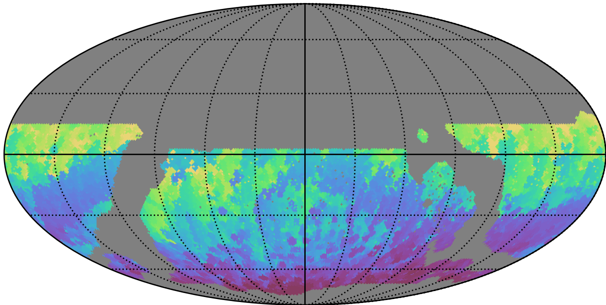
noroll_mjdp365_v3.4_10yrs WFD z band: Min HA
