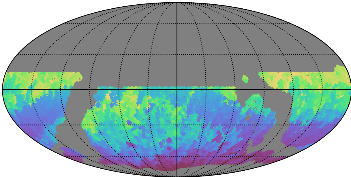
noroll_mjdp365_v3.4_10yrs WFD i band: Min HA
