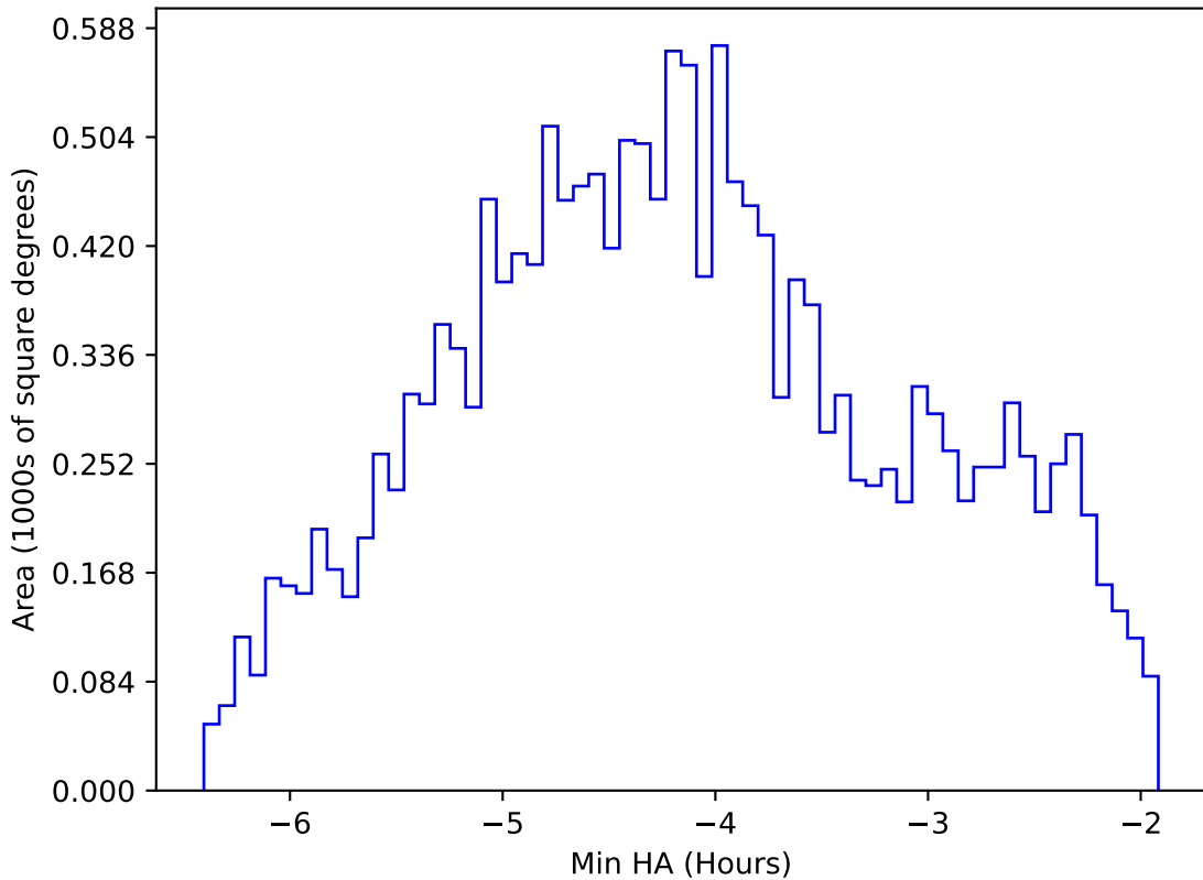
noroll_mjdp365_v3.4_10yrs WFD i band: Min HA
