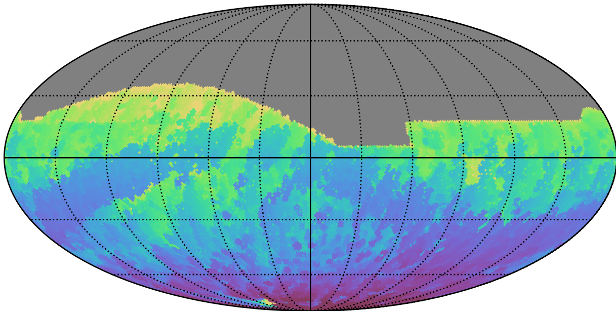
noroll_mjdp365_v3.4_10yrs All sky z band: Min HA
