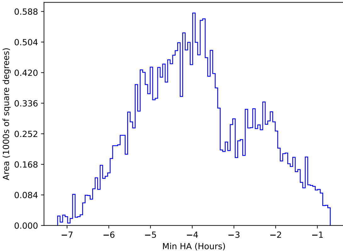
noroll_mjdp365_v3.4_10yrs All sky z band: Min HA
