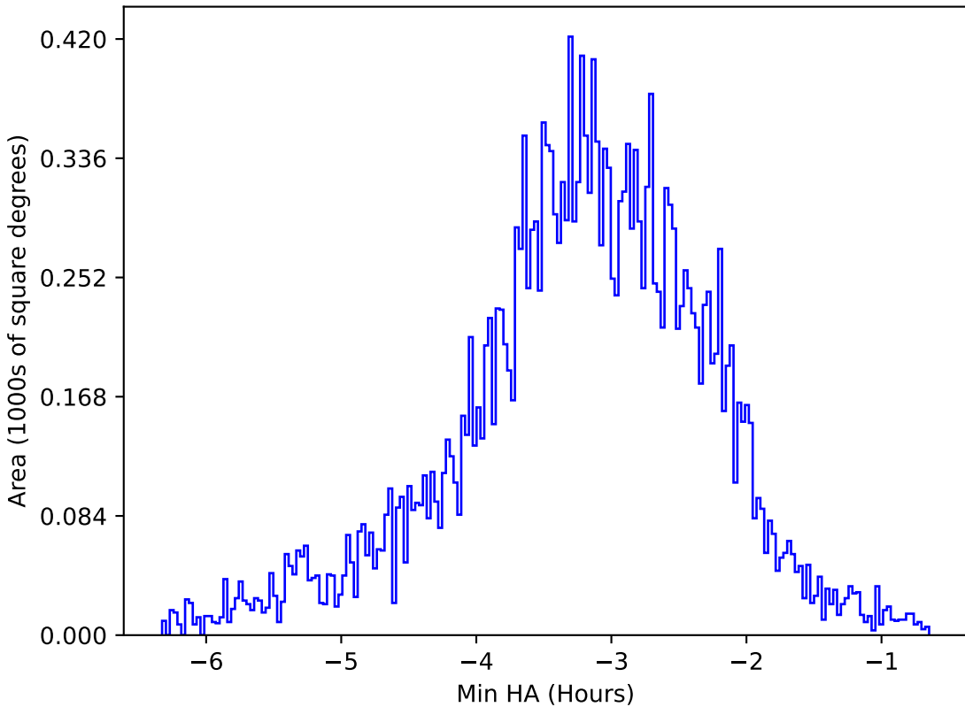
noroll_mjdp365_v3.4_10yrs All sky y band: Min HA
