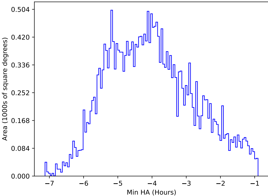
noroll_mjdp365_v3.4_10yrs All sky r band: Min HA
