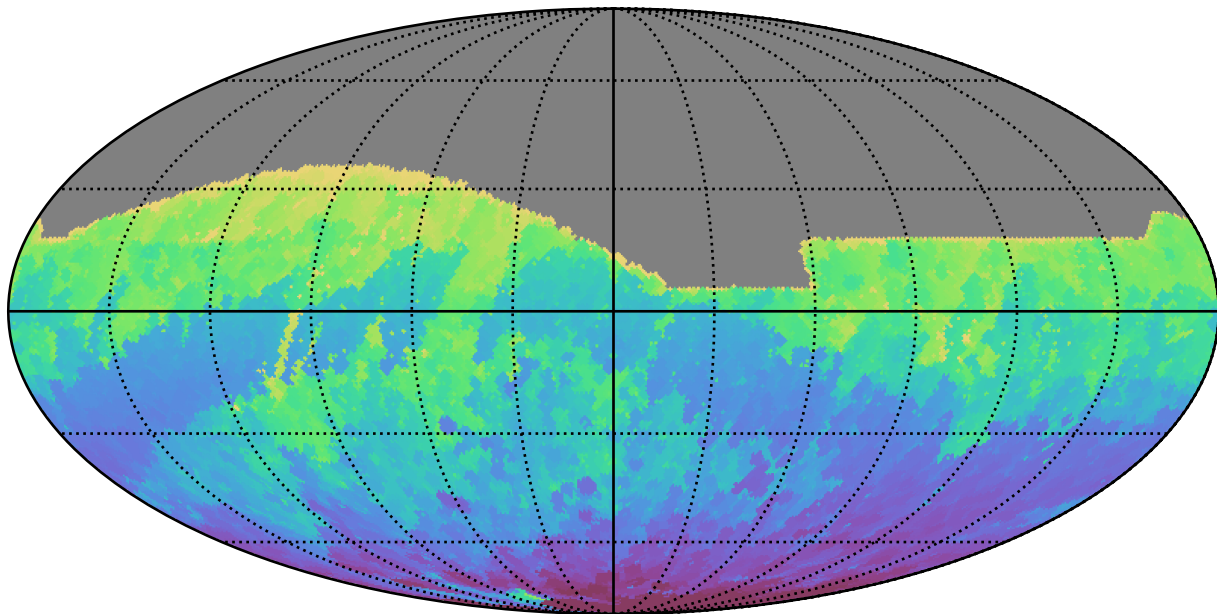
noroll_mjdp365_v3.4_10yrs All sky i band: Min HA
