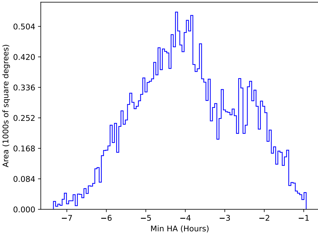
noroll_mjdp365_v3.4_10yrs All sky i band: Min HA
