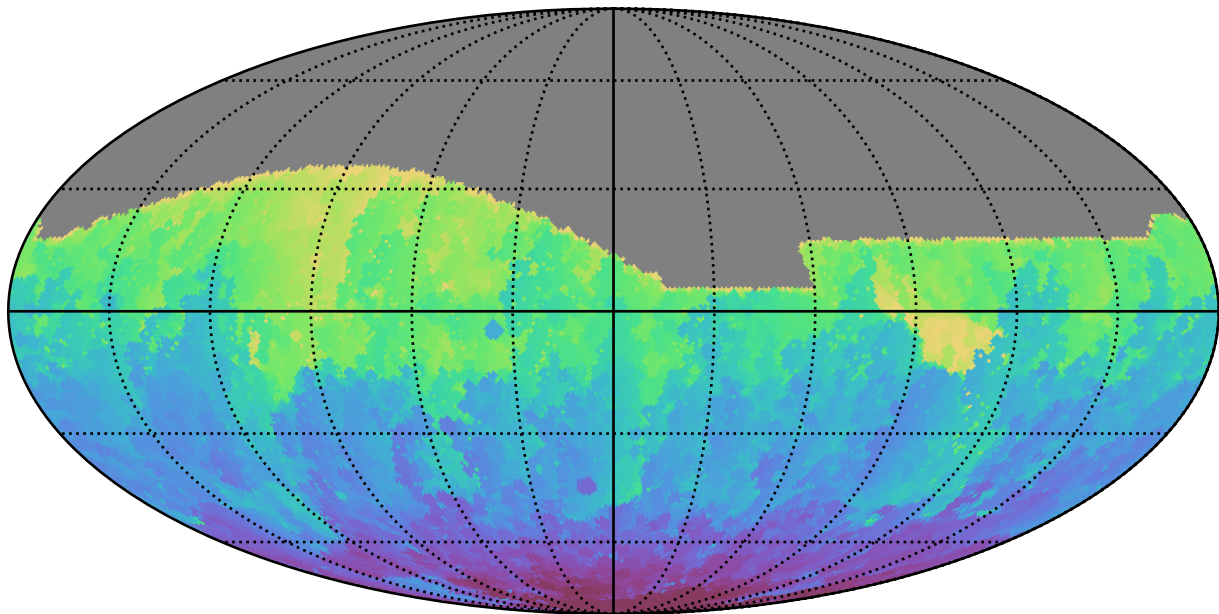
noroll_mjdp365_v3.4_10yrs All sky g band: Min HA
