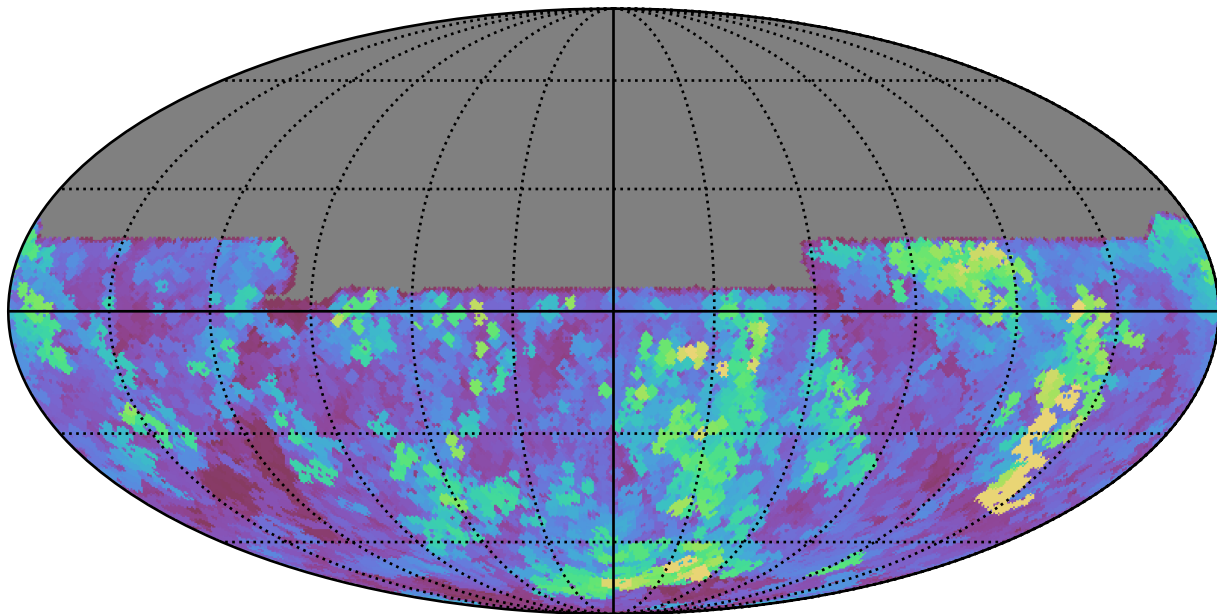
noroll_mjdp365_v3.4_10yrs All sky y band: Max seeingEff
