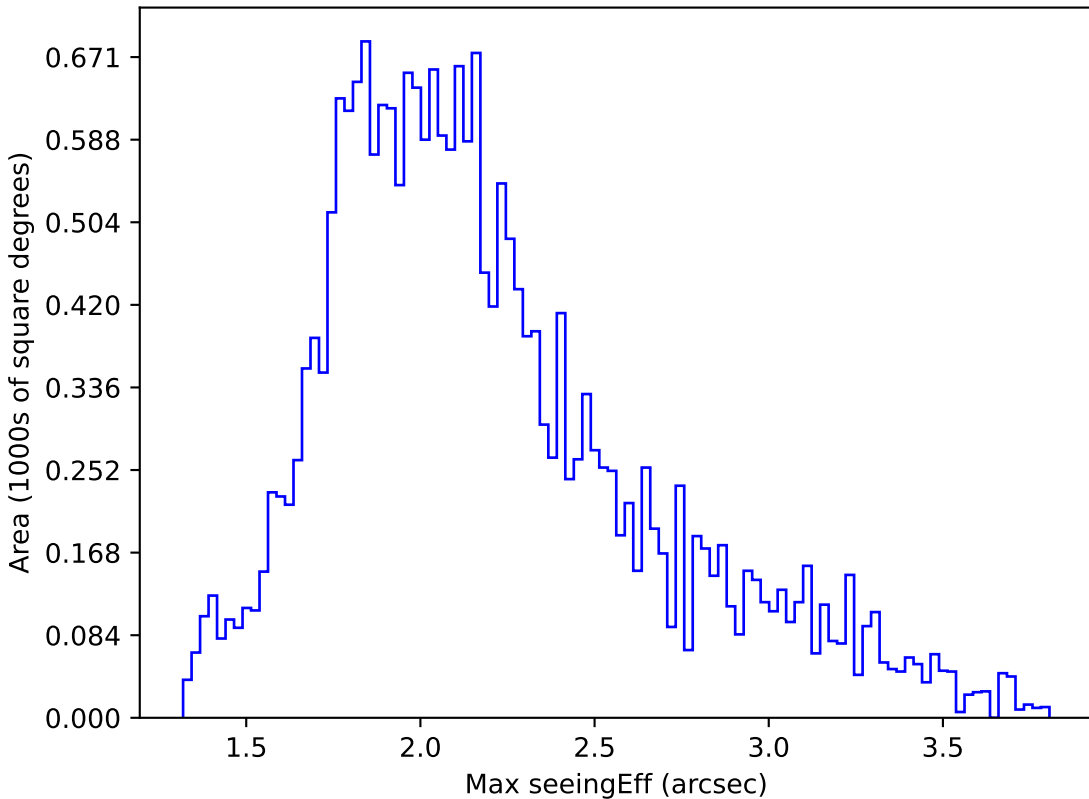
noroll_mjdp365_v3.4_10yrs All sky y band: Max seeingEff
