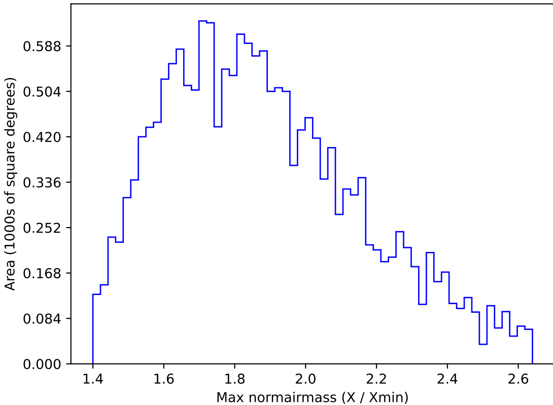
noroll_mjdp365_v3.4_10yrs WFD y band: Max normairmass
