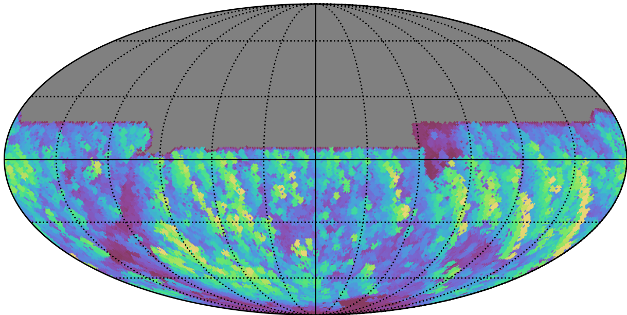
noroll_mjdp365_v3.4_10yrs All sky y band: Max normairmass
