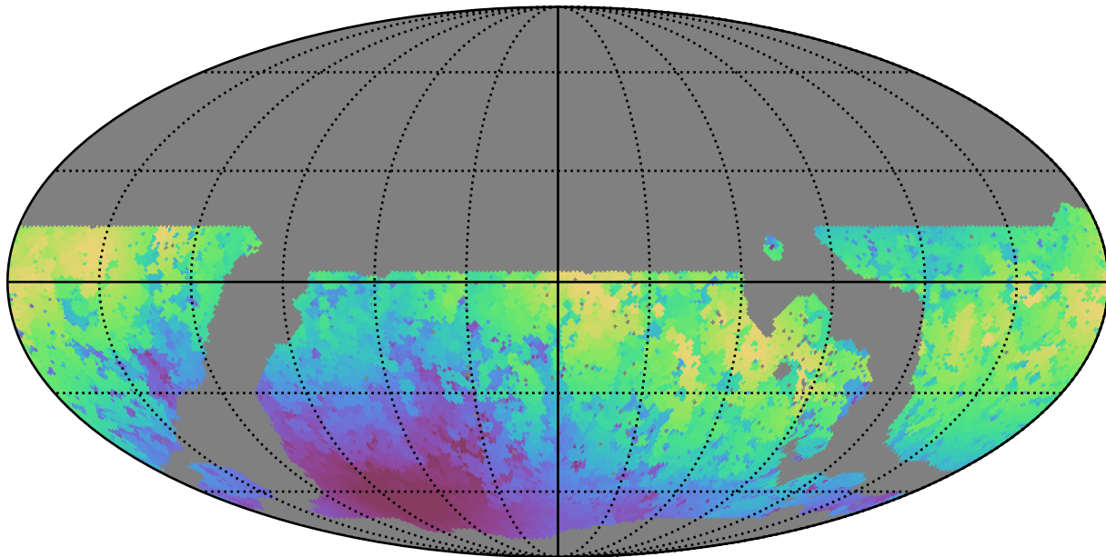
noroll_mjdp365_v3.4_10yrs WFD y band: Max moonDistance
