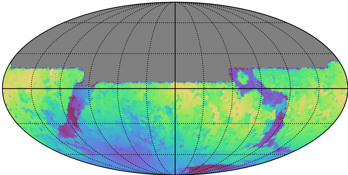
noroll_mjdp365_v3.4_10yrs All sky y band: Max moonDistance
